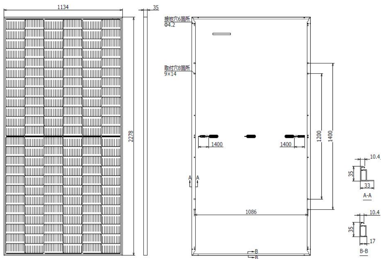
NER144M***B-MD_フレーム厚 35mm
