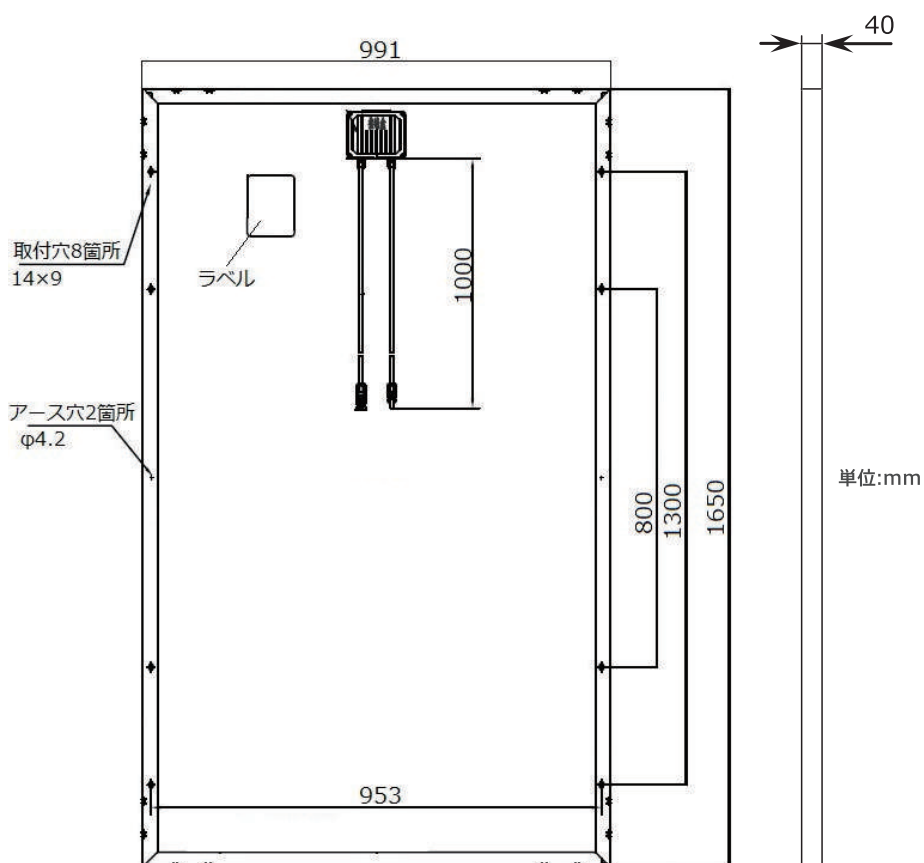
背面図
