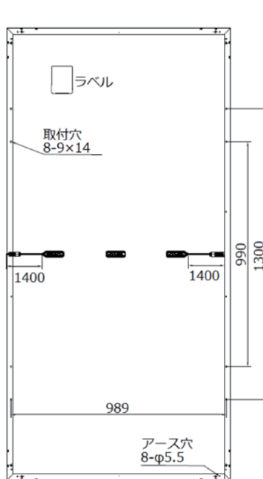
背面図
