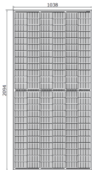
正面図
