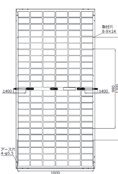
背面図
