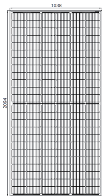
正面図
