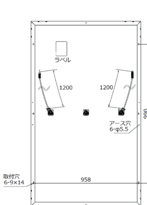
背面図
