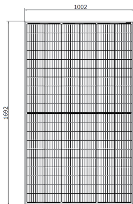
正面図
