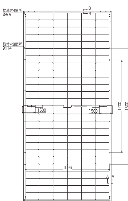
※セル・インターコネクターの配置およびコネクタ・ジャンクションボックスの形状はイメージです
