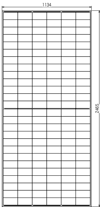
正面図
