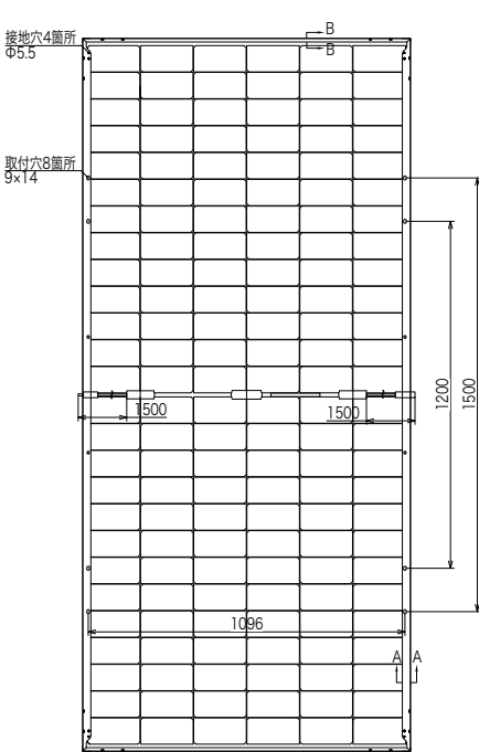
背面図
