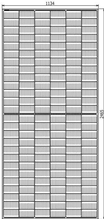
正面図
