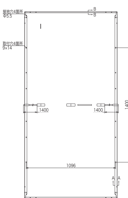
背面図
