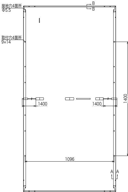
背面図
