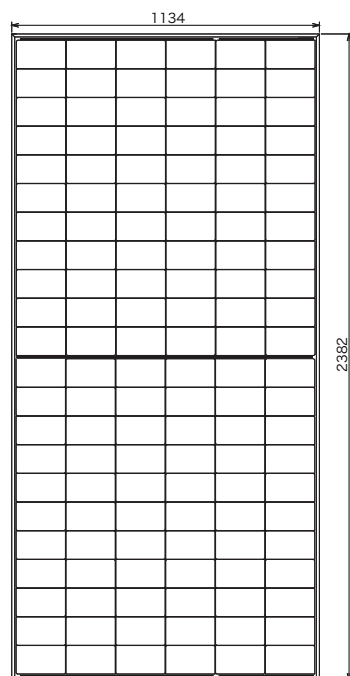
正面図
