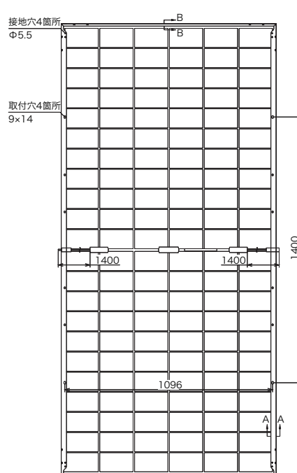
背面図
