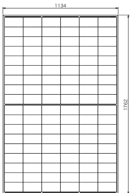
正面図
