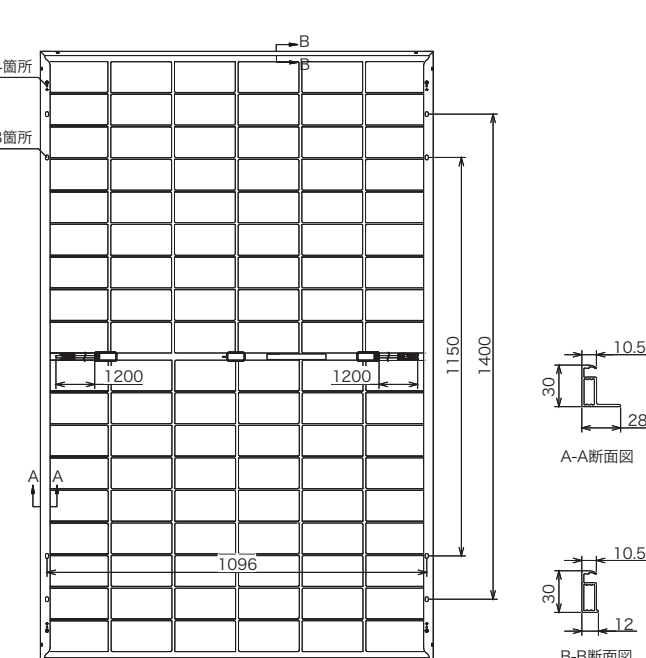
背面図
