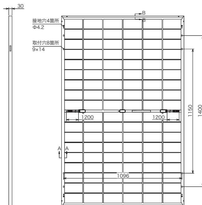
側面図
