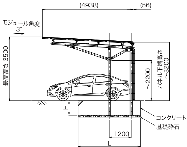
側面図
