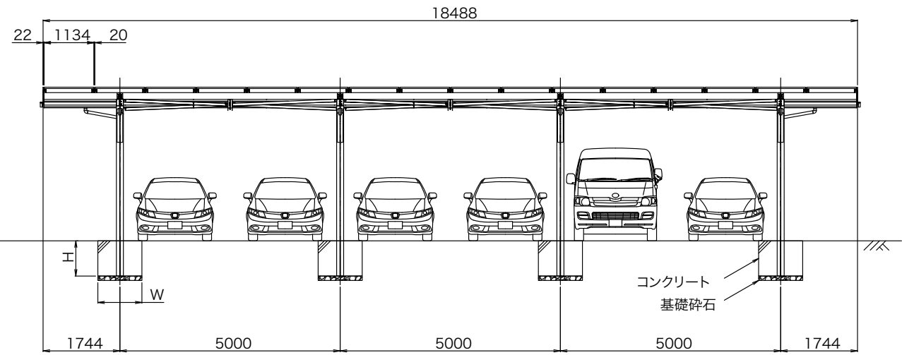
正面図
