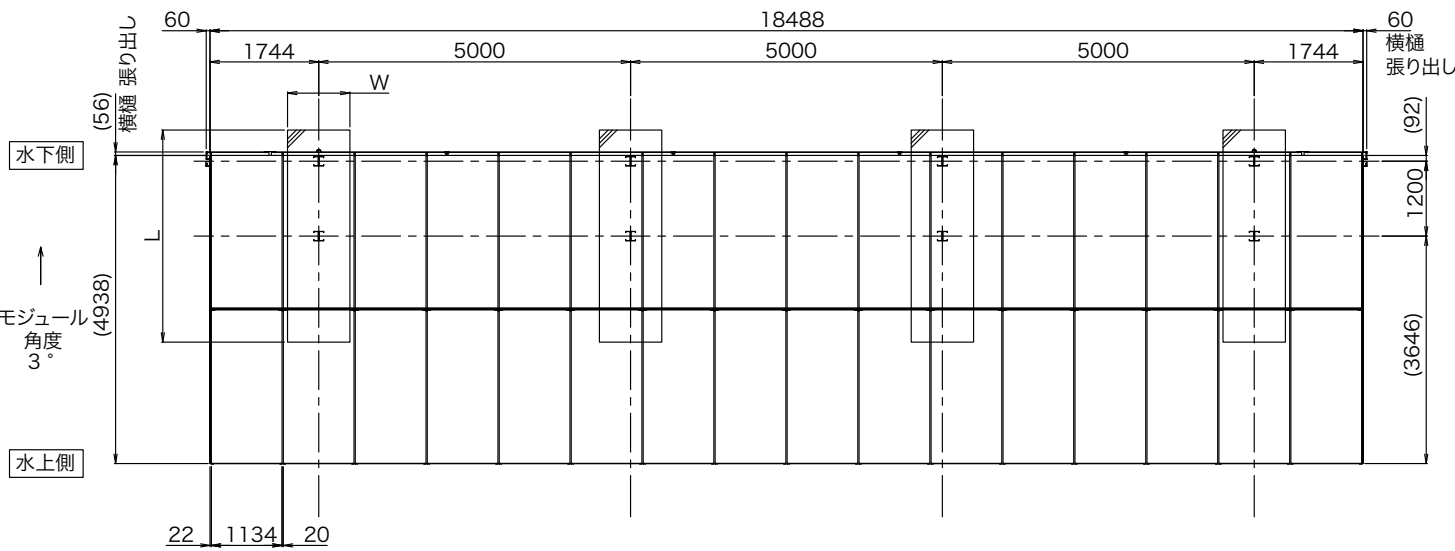
平面図
