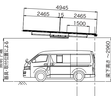
柱間 断面図
