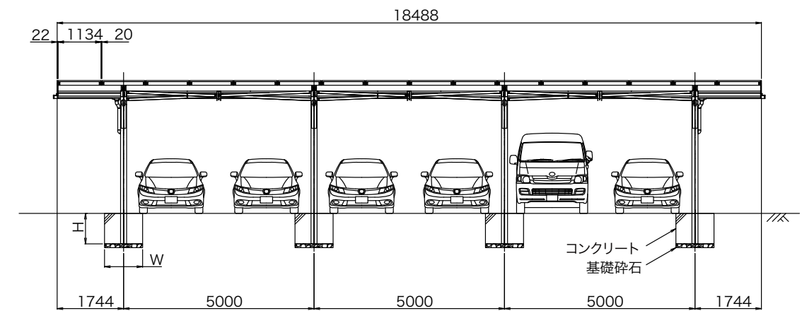
正面図
