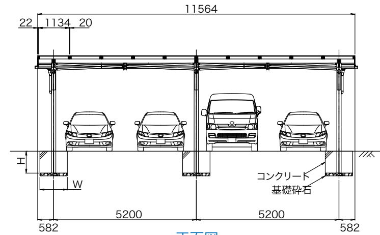
正面図
