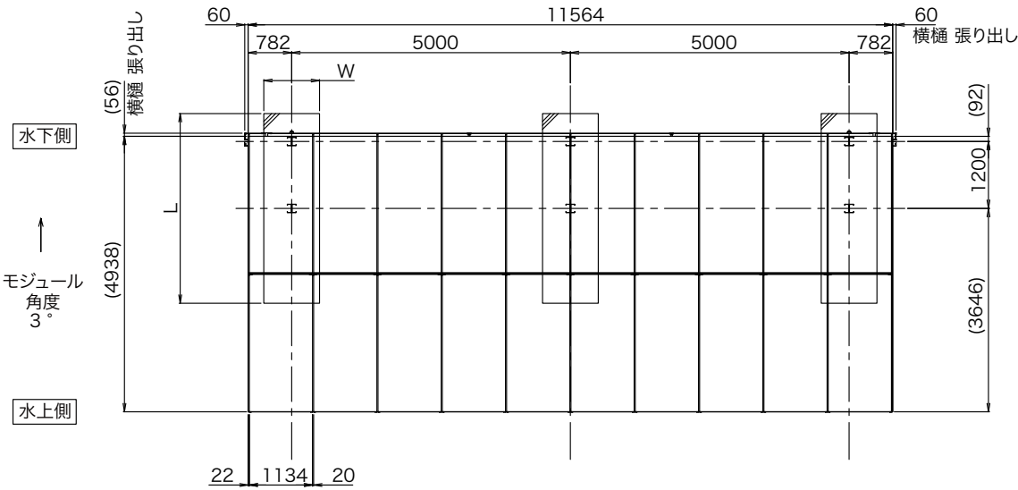
平面図
