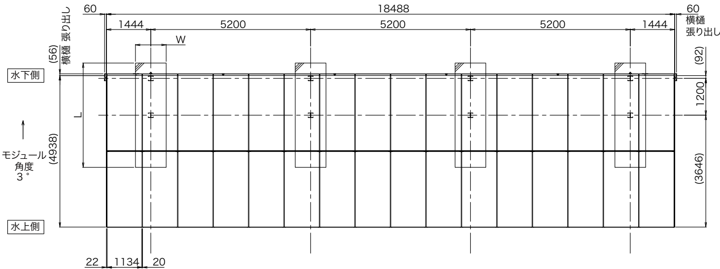
平面図
