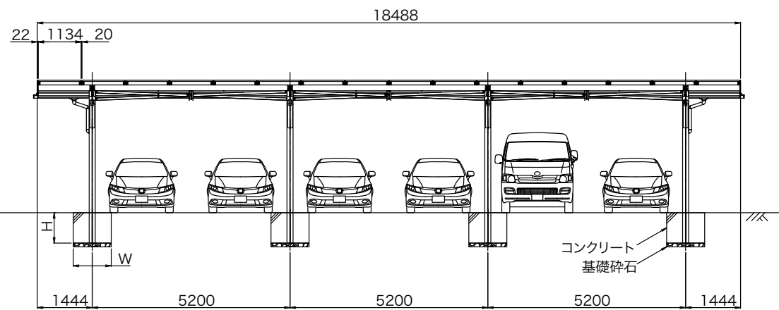
正面図
