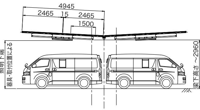
柱間 断面図
