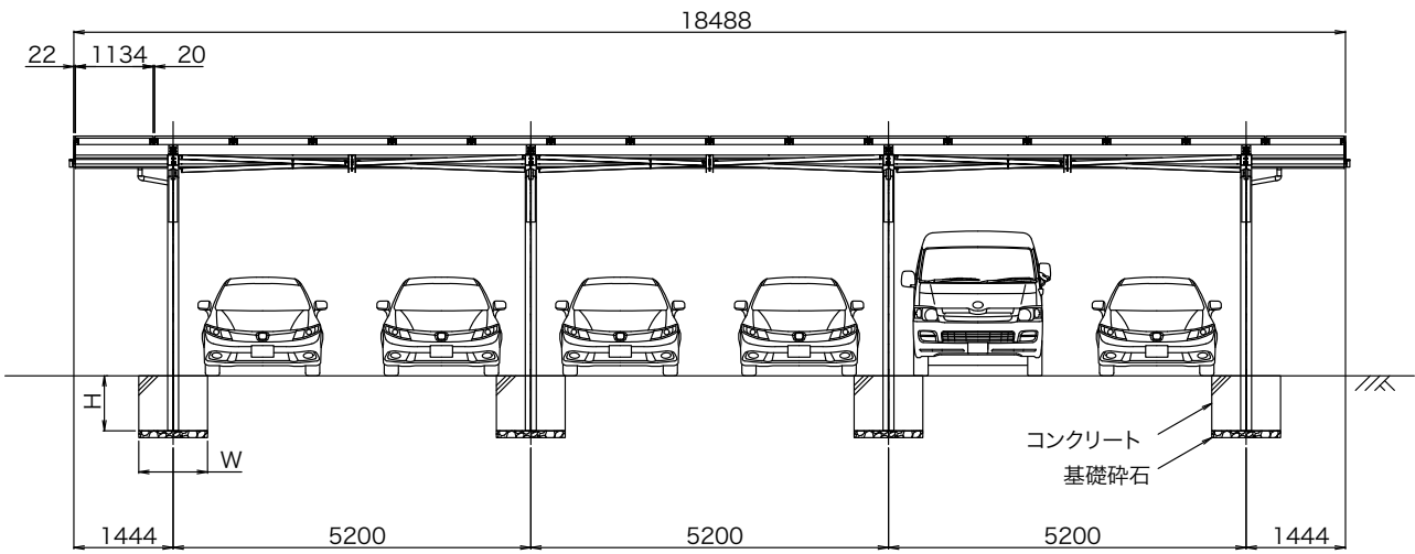
正面図
