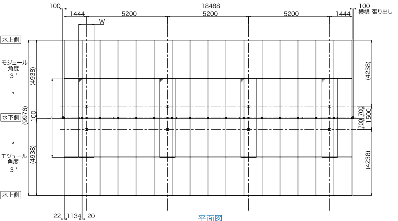
平面図
