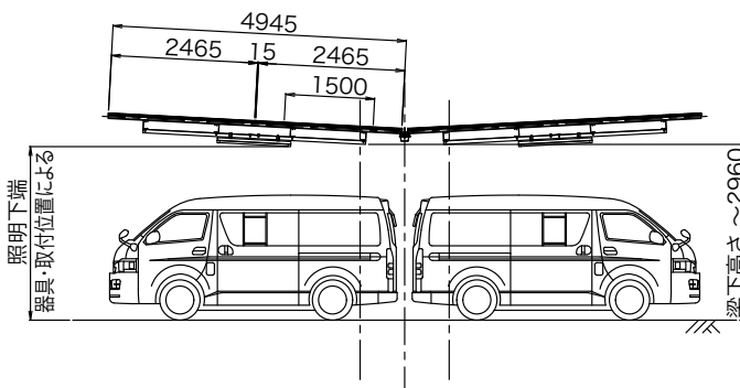
柱間 断面図
