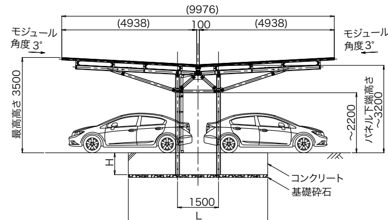
側面図
