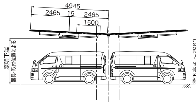
柱間 断面図
