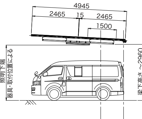
柱間 断面図
