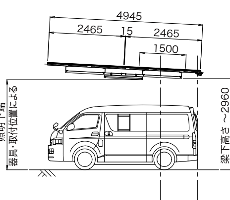
柱間 断面図
