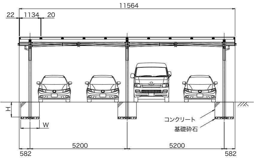
正面図
