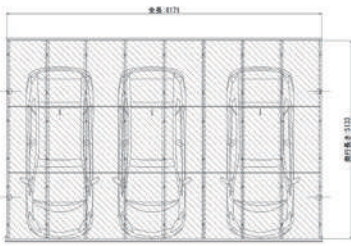
太陽光発電設備（平面図）
