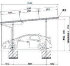
太陽光発電設備（側面図）
