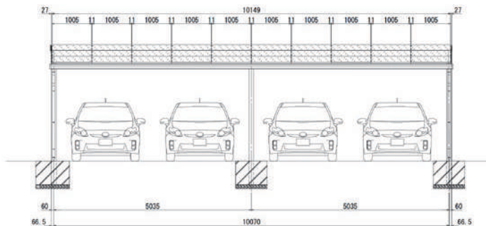
太陽光発電設備（正面図）
