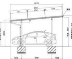
太陽光発電設備（側面図）
