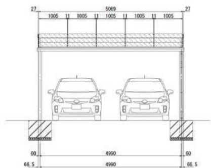
太陽光発電設備（正面図）
