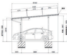
太陽光発電設備（側面図）
