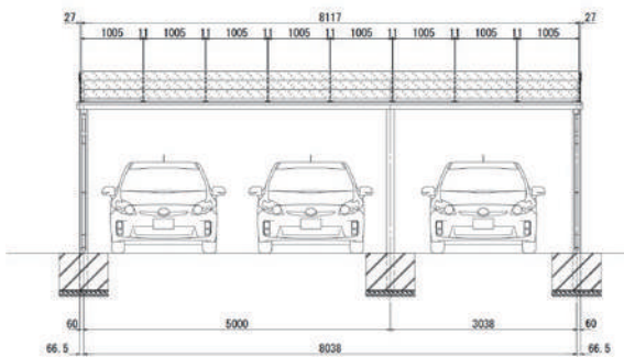
太陽光発電設備（正面図）
