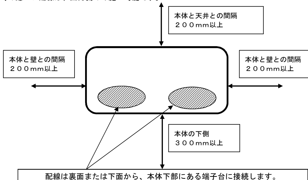
図5-1 壁面取り付け時の周囲との最低スペース
