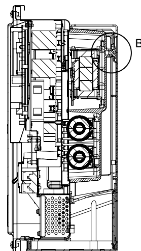
断面図 A-A
