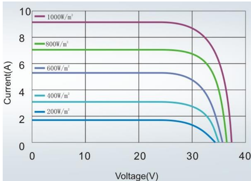
日射量と発電特性の関係 (265W での例)
