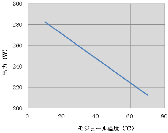
温度と出力の関係 (265W での例)
