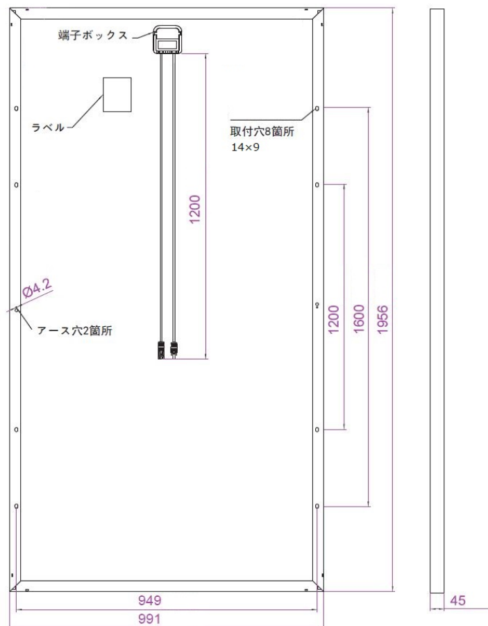
背面図
