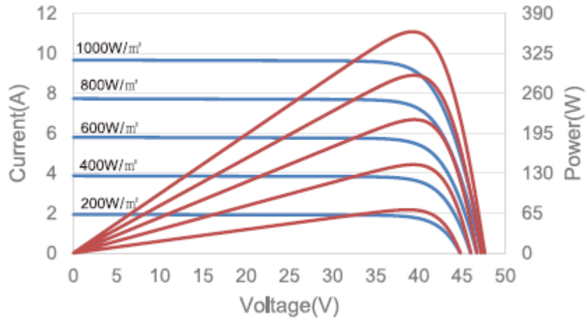
日射量と発電特性の関係 (365W)
