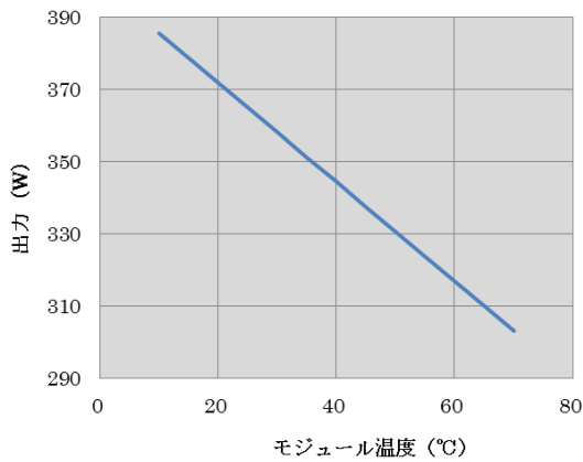
温度と出力の関係 (365W)
