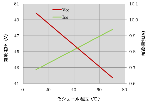
温度と開放電圧、短絡電流の関係 (365W)
