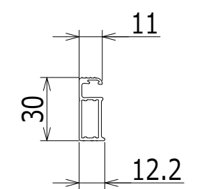
B-B断面図 倍尺 4/1
