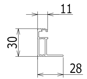
A-A断面図 倍尺 4/1
