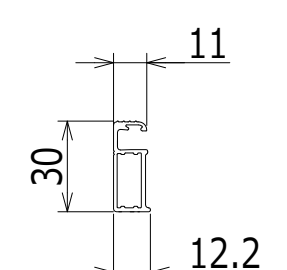
B-B断面図 倍尺 4/1
