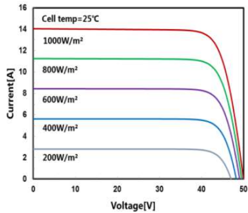
日射量と発電特性の関係
