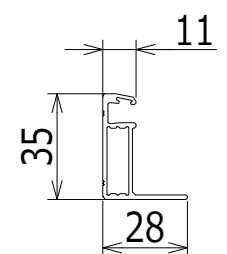
A-A断面図 倍尺 4/1
