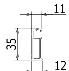
B-B断面図 倍尺 4/1
