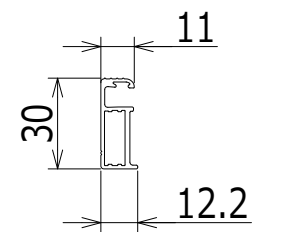
B-B断面図 倍尺 4/1
