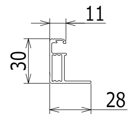
A-A断面図 倍尺 4/1
