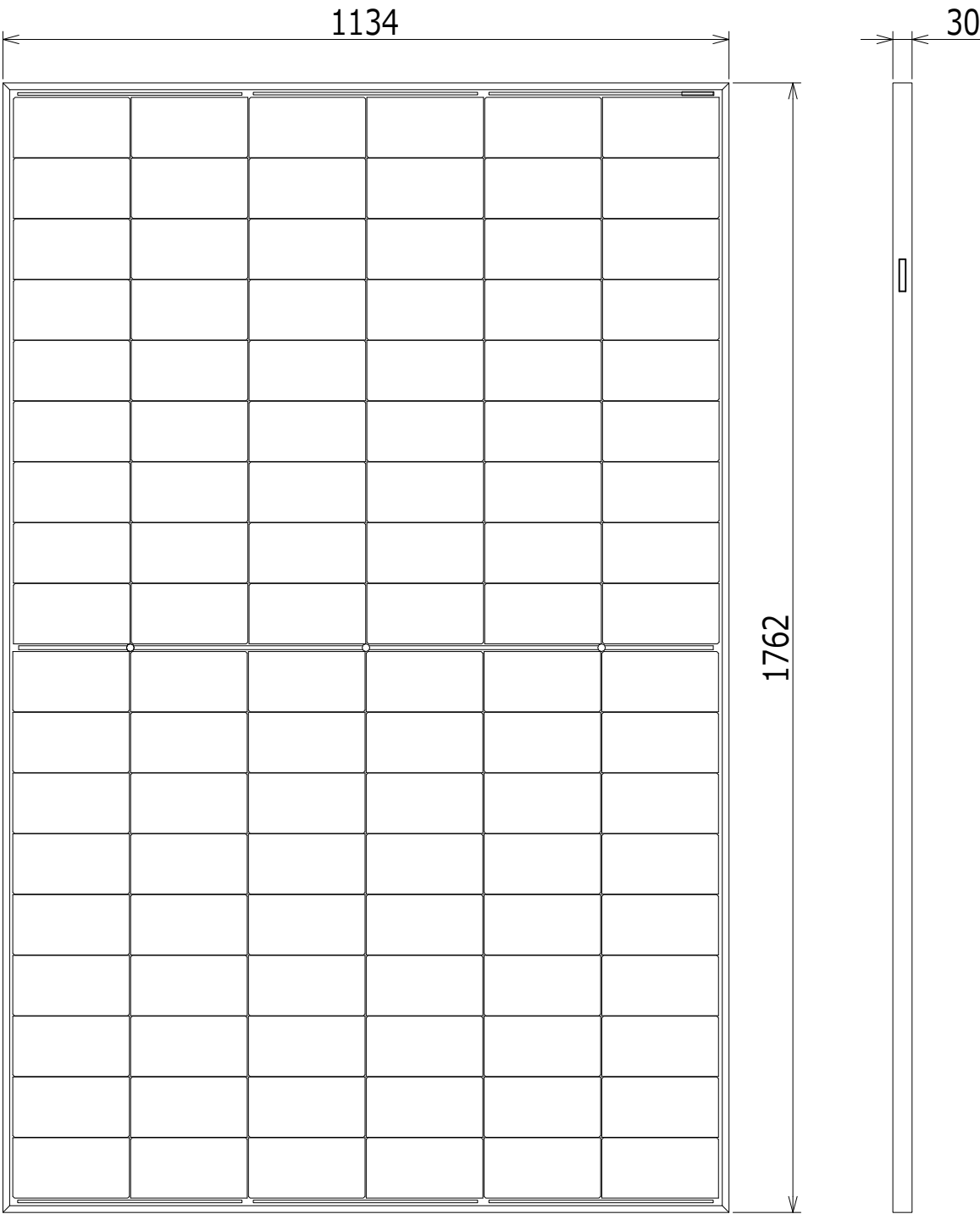
※セル形状・インターコネクターの配置はイメージです
