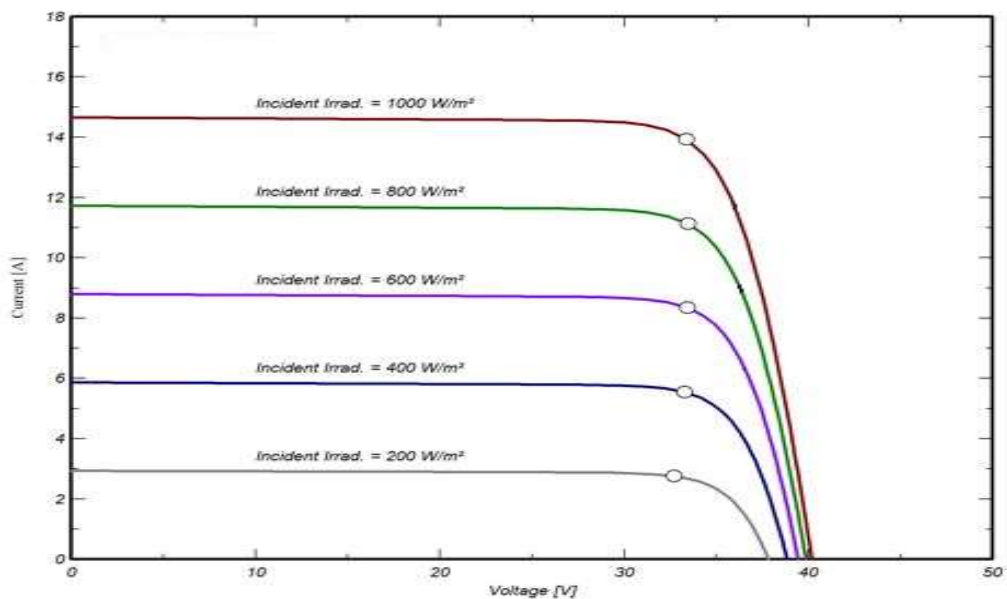
日射量と発電特性の関係
