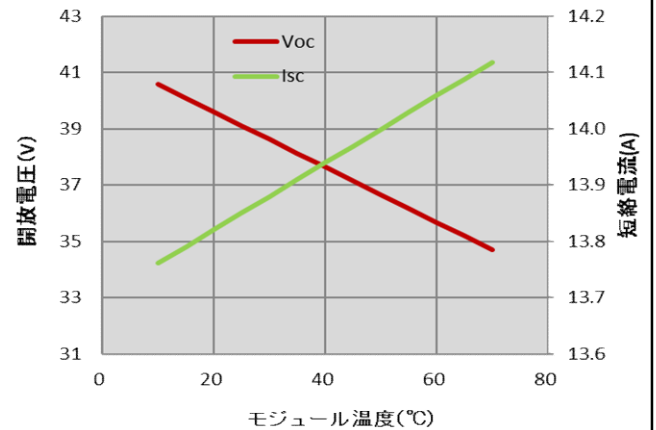
温度と開放電圧、短絡電流の関係
