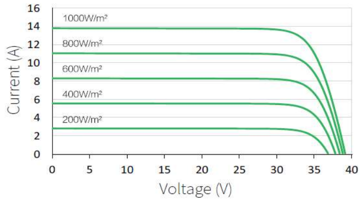
日射量と発電特性の関係
