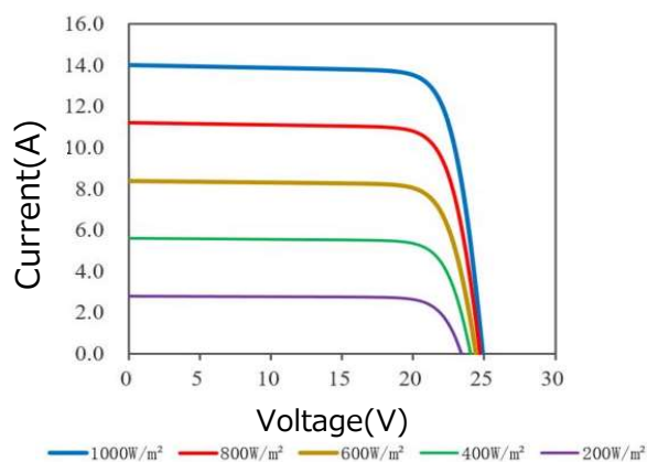
日射量と発電特性の関係
