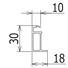
B-B断面図 倍尺 4/1
